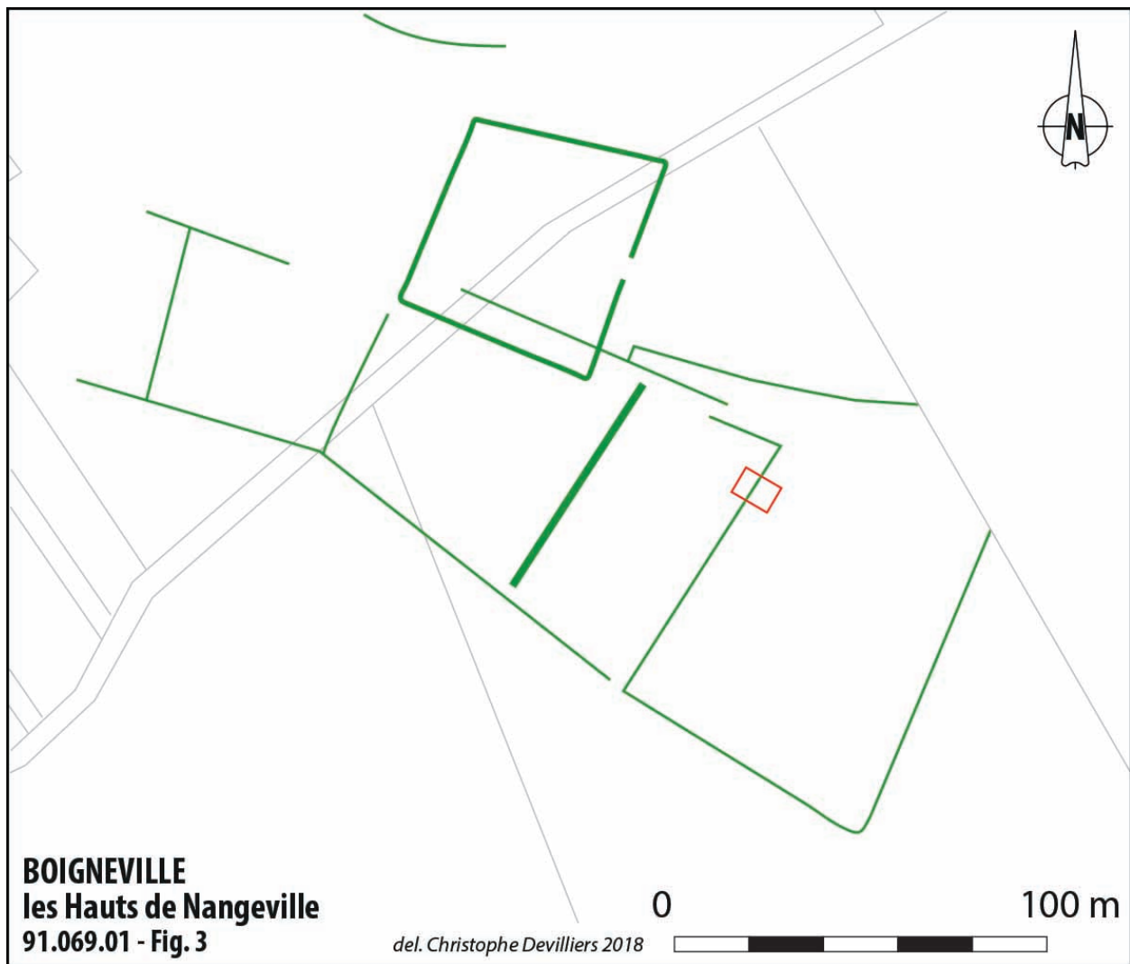
Fig. 3 : plan redressé de l'établissement (DAO Christophe Devilliers, 2018).
